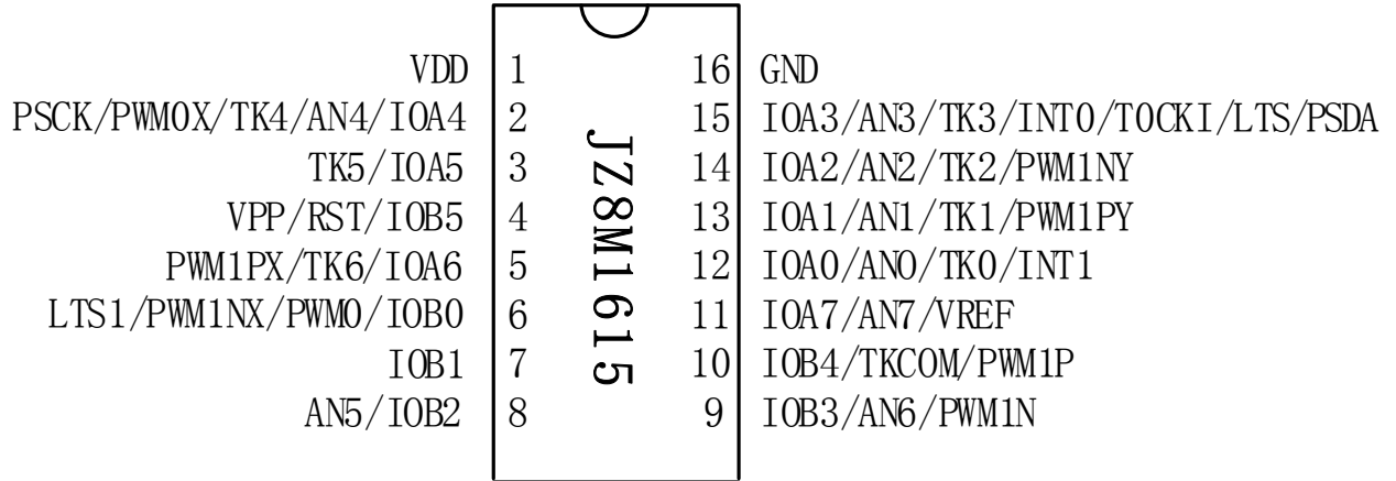
JZ8M1615-16PIN 脚位图
