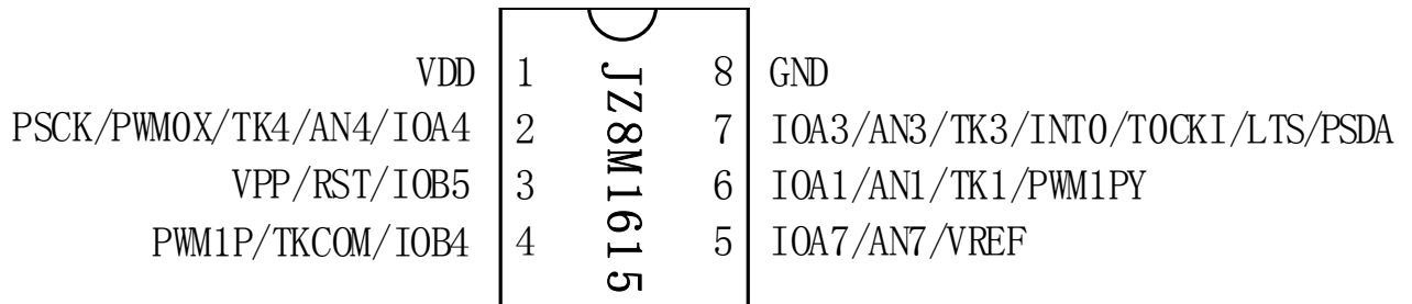
JZ8M1615-8PIN 脚位图
