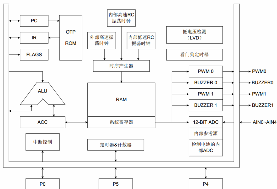
系统结构框图
