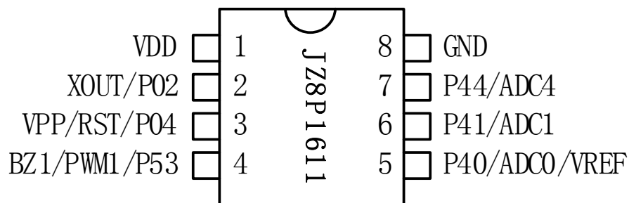
JZ8P1611-8PIN 脚位图
