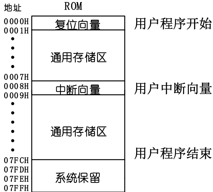
程序存储器区结构图
