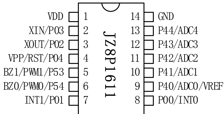
JZ8P1611-14PIN 脚位图
